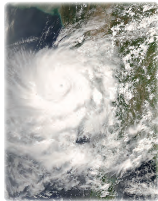
Ciclonul Nargi înainte de a pătrunde pe uscat
